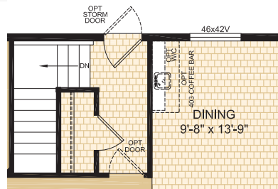
Optional Foundation
